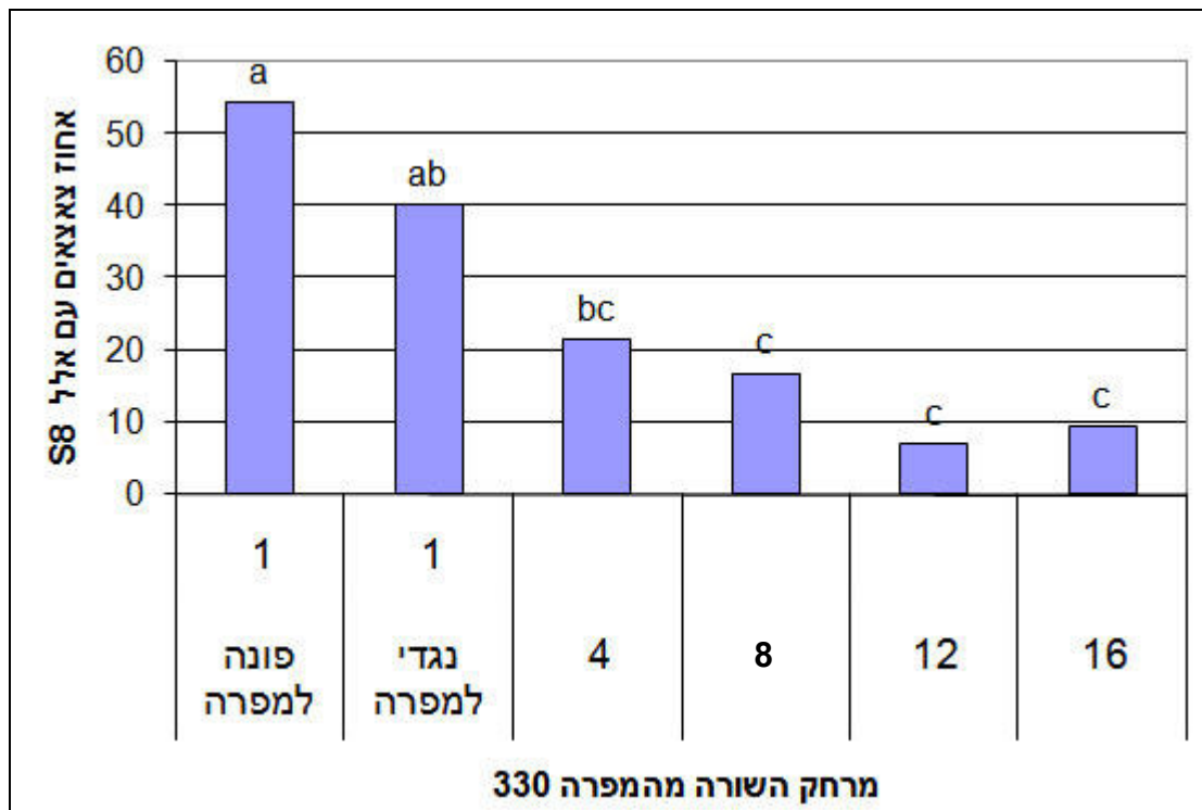
איור 8. אחוז צאצאי 333 בעלי אלל S8 (מהזן 330), ראש פינה 2008.
