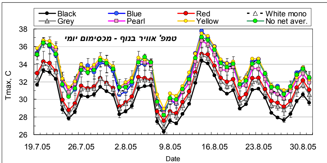
איור 1. טמפרטורות מכסימום יומיות בנוף העץ תחת הרשתות ובביקורת, ביולי-אוגוסט 2004 ו-2005. ממוצע 3 יחידות הובו לטיפול. ההובואים נתלו בגובה 1.5 מ' מהקרקע, בתוך נוף העץ.
