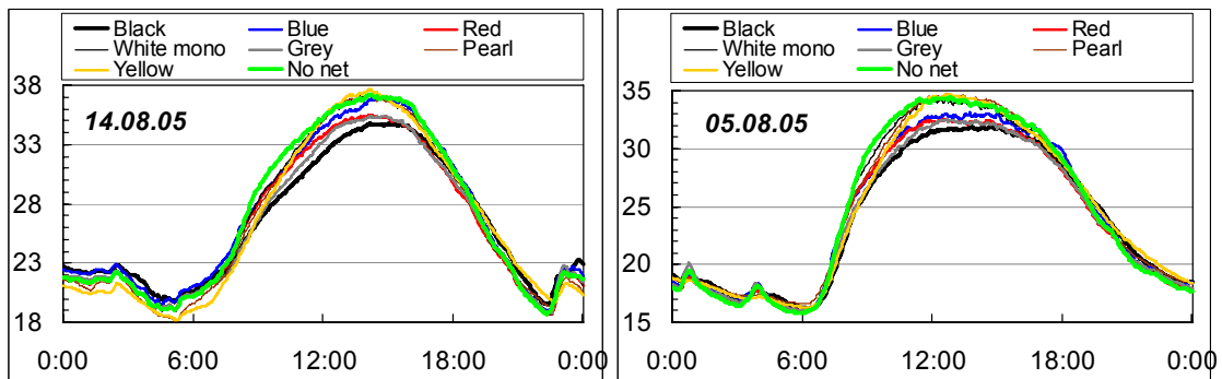
איור 2. עקום יומי של טמפ' האוויר בנוף תחת הרשתות והביקורת ביום של טמפ' ממוצעת לעונה (5.8.05) וביום חם מהממוצע (14.8.05). כל עקום הוא ממוצע של 3 יחידות הובו לטיפול.
